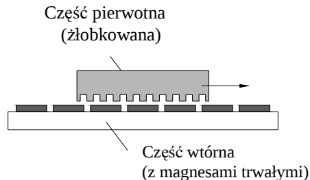
Rys.6. Schemat budowy silnika synchronicznego
